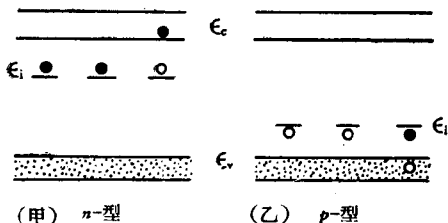
图 26-9. 半导体中的杂质能級: (甲) n -型半导体的給电子能級; (乙) p -型半导体的受电子能級
