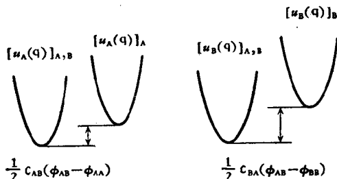
图 37-1. 正规溶体和单组分晶体中分子 A 和 B 的位能函数的对比
