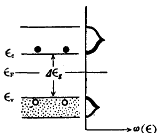
图 26-8. 半导体的能帶模型
