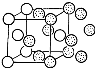
图 36-3. 汞晶体的立方最密堆积结构 与其中汞原子的配位
