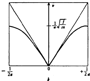
图 35-4. 在一个无限的点阵结构中弹性波的频率随传播常数递变的情况
