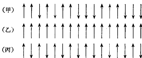
图 36-5. 顺磁物质的自旋取向分布的示意: (甲)顺磁物质在居里点以上时的无序构型; (乙)铁磁物质在居里点以下时的有序构型, (丙)反铁磁物质在居里点以下时的有序构型
