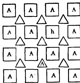
图 36-8. 弗伦克尔缺陷模型
