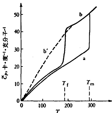
图 23-4. 甘油的比热曲线
