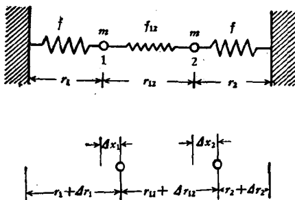
图 10-3. 单維偶合振子体系 系统的位能函数为
