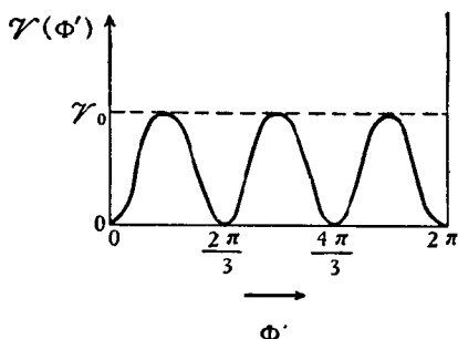
图 23-8. 乙烷分子中两个甲基內旋轉的位能函数
