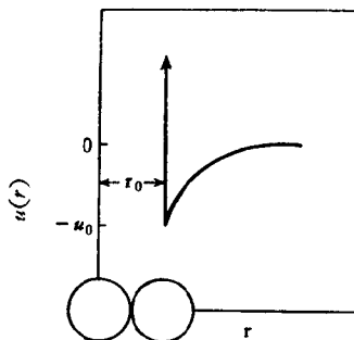
图 30-3. 范德华气体中分子间相互作用的位能函数
