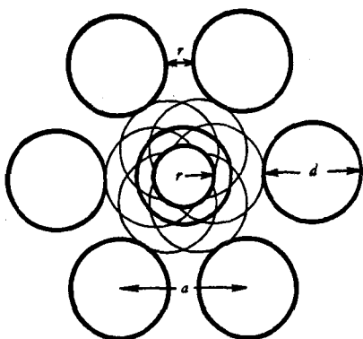
图 33-1. 液体中分子的囚胞
