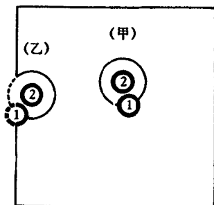
图 30-2. 分子对 1-2 在气体容器中的两种处境: (甲) 分子 2 在容器深处; (乙) 分子 2 接近器壁
