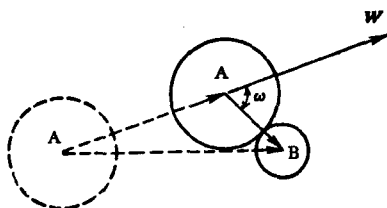
图 19-4. 分子 A 和 B 碰撞时相对速度向量 \vec{W} 和連接分子中心的向量 \vec{AB} 以及它們之間的交角 \omega
