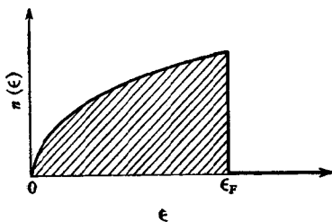
图 26-3. 电子气在 0^\circ\text{K} 下的能级分布
