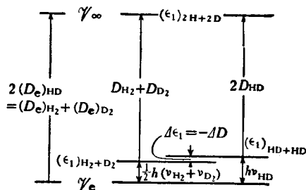
图 16-1. 反应物 ( \text{H}_2 + \text{D}_2 ) 和生成物 ( \text{HD} + \text{HD} ) 以及 ( \text{H} + \text{H} + \text{D} + \text{D} ) 等基态能級間的关系图
