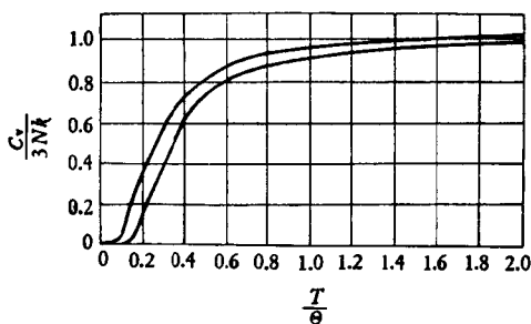
图 6-2. 爱因斯坦晶体(下)和德拜晶体(上)的比热曲线
