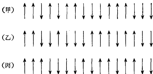
图 36-9. 属于单维自旋体系某一个取向组合的若干个取向排列
