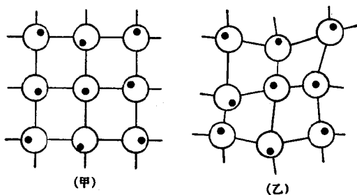
图 23-5. 结构特点和运动形式的示意图:
