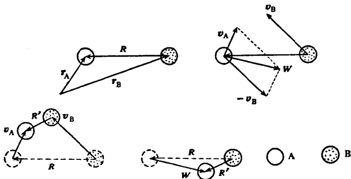
图 19-3. 分子 A 和 B 的相对速度
