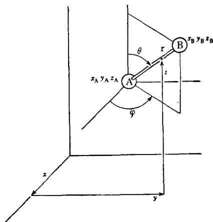
图 9-2. 双原子分子的坐标 x, y, z 和 r, \theta, \varphi
