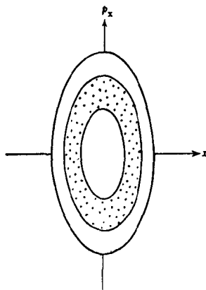
图 8-1. 单維簡諧振子的三个椭圆相軌道: 它們的能量各为 h\nu, 2h\nu 和 3h\nu .
