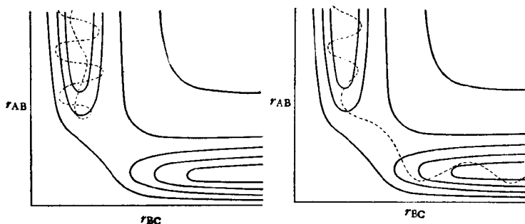
图 20-3. 反应物系中原子 A 与分子(B—C)的碰撞
