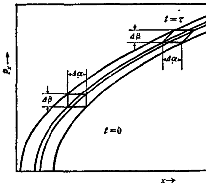
图 7-1. 相体积不变原理的例示
