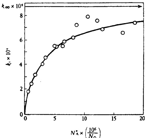
图 21-2. 二甲醚在 777.2° K 下的分解反应及其速度常数 k_r 对浓度 N_A^* 的图线
