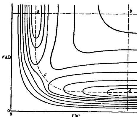
图 20-1. 直线反应物系的位能面及其反应坐标和过渡状态
