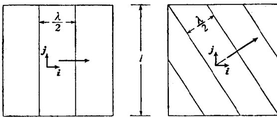
图 26-1. 立方体空腔内的两个驻波
