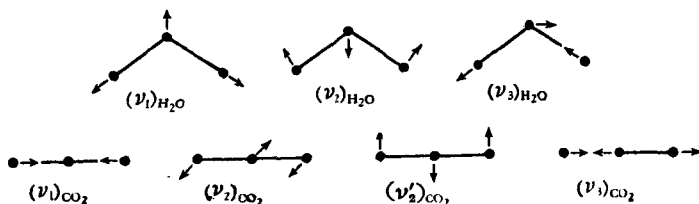
图 10-5. \text{H}_2\text{O} 和 \text{CO}_2 分子的简正振动方式
