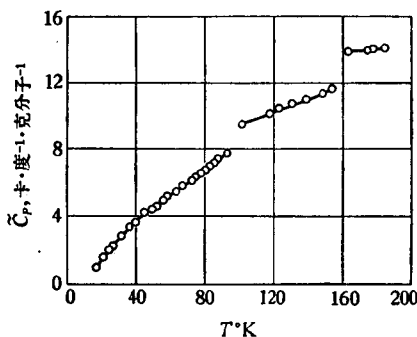
图 23-1. 氯化氢的比热曲线(16—188.1°K)
