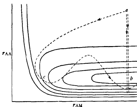
图21-1. 反应物系(A+A+M)的位能面
