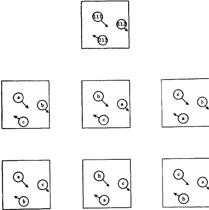
图 3-2. 离域子体系的微观状态示意图
