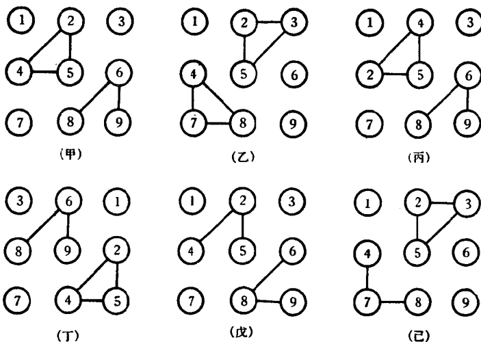
图 31-2. 九分子体系的某三个集团排列及其所隶属的两个集团组合
