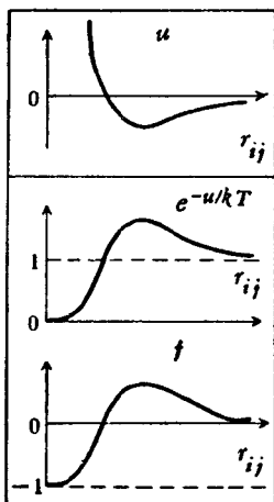
图 30-1. 一对分子的相互作用 給出的函数 u(r_{ij}) , e^{-u(r_{ij})/kT} 和 f_{ij}
