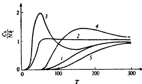
图 9-6. 氢气的轉动比热曲线示意图
