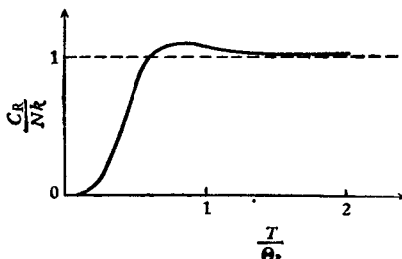
图 9-4 异核双原子分子气体的转动比热曲线示意图
