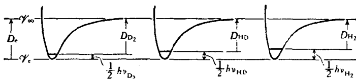
图 17-1. 双原子分子 H_2 , D_2 和 HD 的位能函数
