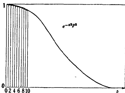
图 6-1. 级数 \sum_{p=1}^{\infty} e^{-\alpha^2 p^2} 和定积分 \int_0^{\infty} e^{-\alpha^2 p^2} dp 的关系
