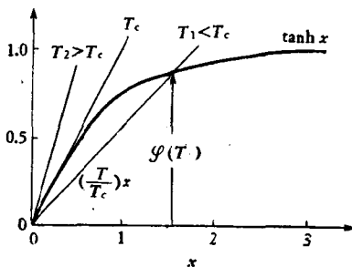
图 38-7. 有序度方程 \left(\frac{T}{T_c}\right) x = \tanh x 的图解
