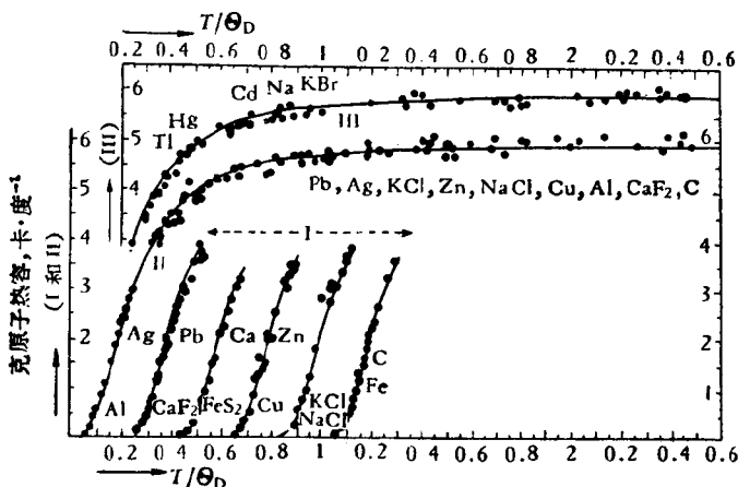
图 35-2. 十八种晶体的比热实验值与德拜理论曲线
