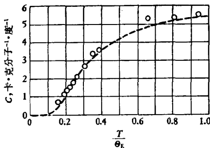
图 35-1. 金刚石的比热数据和按照爱因斯坦模型計算出来的比热曲綫(比热曲綫的爱因斯坦溫度 \Theta_E = 1320^\circ\text{K} )
