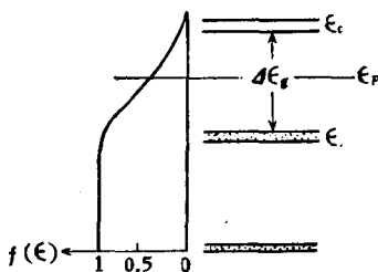
圖 26-7. 絕緣體能帶的簡化模型和電子分布情況
