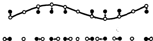
图 35-5. 单維晶体中一个駐波的示意图
