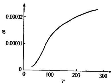
图 24-2. 铝的线膨胀系数曲线
