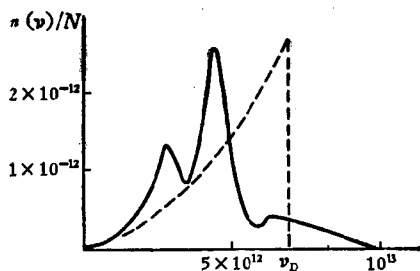
图 35-7. NaCl 晶体的频率分布函数: 点阵结构模型 (实线) 和德拜模型 (虚线)
