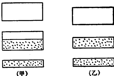
图 26-6. 固体的能带构造和电子结构： (甲)金属；(乙)絕緣体和半导体
