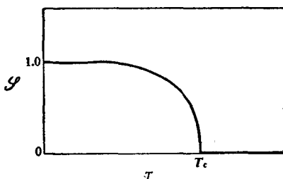
图 38-8. \beta -黃銅的有序度随温度递变的情况
