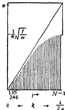
图 35-6. 单維晶体的頻率和传播常数
