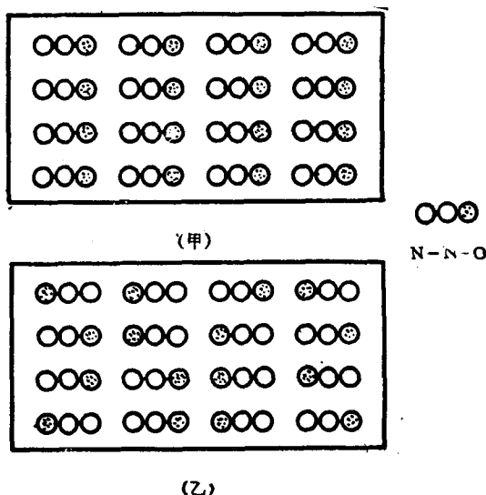
图 36-4. \text{N}_2\text{O} 晶体中直线分子 \text{NNO} 的取向无序: (甲)有序取向构型; (乙)无序取向构型
