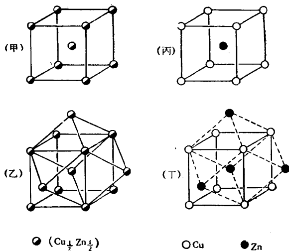
图 38-6. 组成为 \text{CuZn} 的 \beta -黄铜：(甲)无序结构的立方体心单位；(乙)无序结构的三方素单位；(丙)超结构的立方素单位；(丁)超结构没有三方素单位
