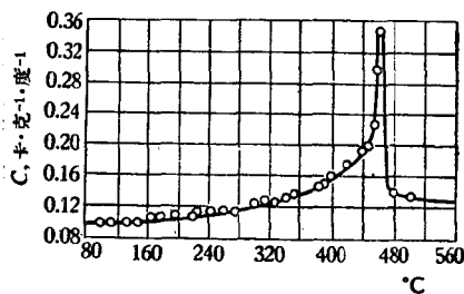
图 38-9. \beta -黄铜的实验比热曲线(样品的组成相当于化学式 \text{Cu}_{0.51}\text{Zn}_{0.49} )
