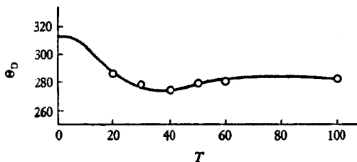
图 35-8. NaCl 晶体在低温区间内给出的德拜温度: 曲线是比热实验值给出的, 而小圆圈是点阵结构模型的计算值给出的
