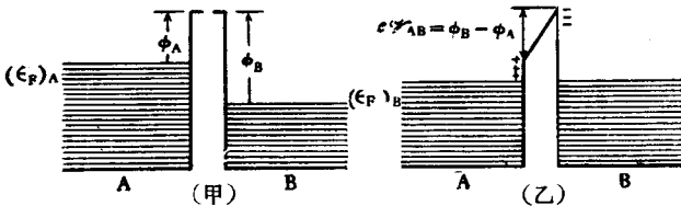
图 26-5. 金属 A 和 B 的接触与其中电子气的平衡: (甲) 电子气达成平衡之前; (乙) 电子气达成平衡之后
