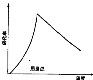
图 36-6. 反铁磁物质的磁化率随温度递变的情况
