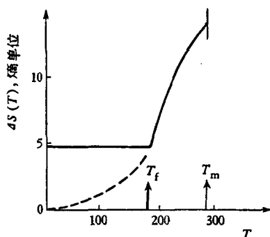
图 23-6. 在温度 T^\circ\text{K} 下超冷液态和玻璃态甘油 超过晶态甘油的额外熵值 \Delta S(T)
