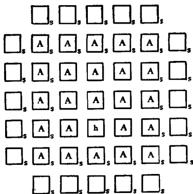
图 36-7. 萧脱基缺陷模型
