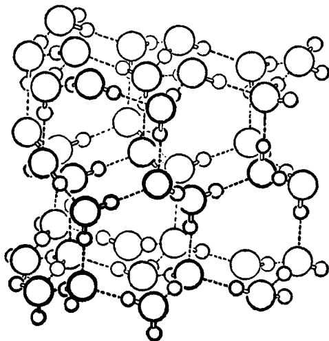
图 23-2. 冰的结构
