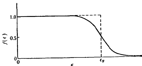
图 26-4. 电子气在 T^\circ\text{K} 的费密分布密度函数
