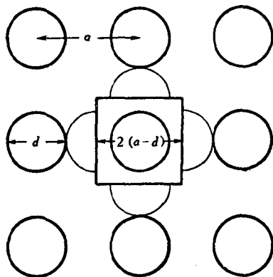
图 33-2. 按简单立方点阵聚集在一起的液体分子和分子的自由体积
