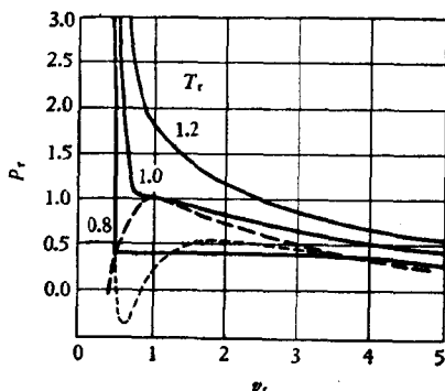
图 32-1. 簡化范德华方程的图綫
