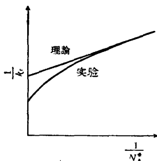
图 21-4. 单分子反应的图綫
