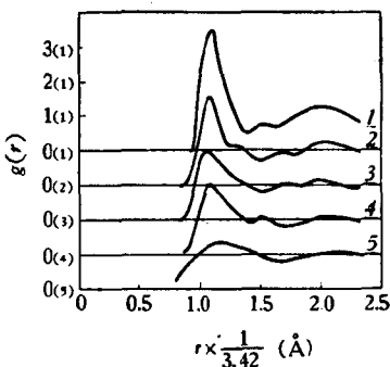
图 34-1. 液态氩在五个不同温度下给出的径向分布函数的实验曲线, 给出曲线 1、2、3、4 和 5 的温度各为 84.4, 91.8, 126.7, 144.1 和 149.3°K。
