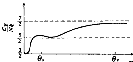
图 9-5. 双原子分子气体的比热曲线示意图
