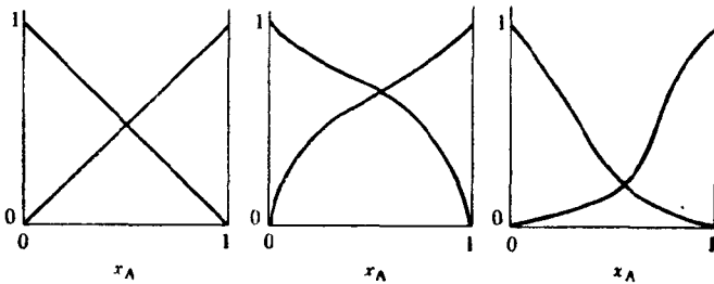
图 38-1. 正規溶体与喇烏耳定律: (甲) \phi = 0 ; (乙) \phi > 0 ; (丙) \phi < 0 .
