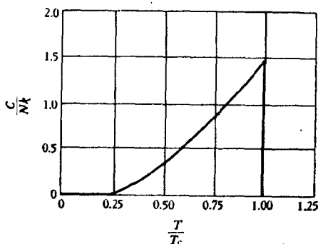
图 38-10. \beta -黄铜的理论比热曲线
