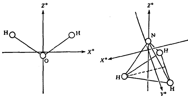
图 10-1. \text{H}_2\text{O} 和 \text{NH}_3 分子以及它們的主軸系
