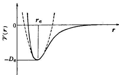
图 9-1. 双原子分子的能量曲线(实线)和简谐振子的位能抛物线(虚线)
