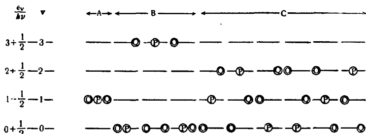
图 3-1. 总振动能 E = \frac{9}{2} h\nu 和振动物子定点 O, P, Q 附近的三个单維振子組成的体系有十个微观状态，它們体现了三种不同的分布 A, B 和 C
