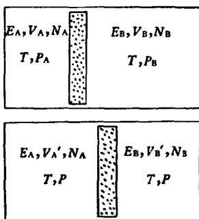
图 14-1. 两个气体通过活塞的滑动达成压力平衡
