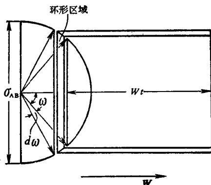
图 19-5. 半径为 \sigma_{AB} 的球面和相当于交角间隔 \omega \rightarrow \omega + d\omega 的环形区域
