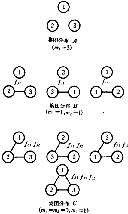
图 31-1. 三分子体系的八个集团排列和三个集团分布
