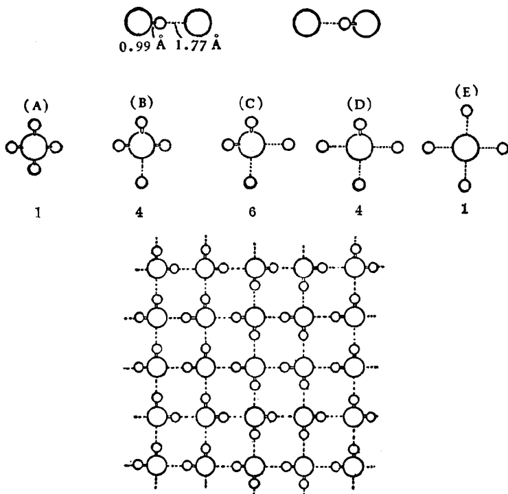
图 23-3. 冰中H原子在O原子周围的分布方式: (上)每对O原子間H原子的分布方式;(中)每个O原子 周围四个H原子的分布方式;(下)冰中H原子空間分布 的一个无序构型
