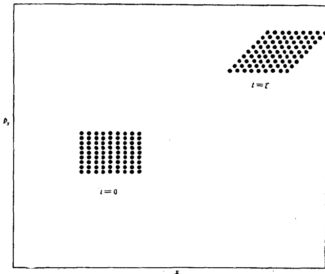
图 7-2. 相点密度不变原理的示意
