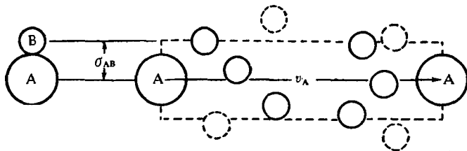
图 19-2. 速度为 v_A 的A分子在单位時間內以有效半径 \sigma_{AB} 在气体中扫过一个体积为 (\pi\sigma_{AB}^2 v_A) 的区域
