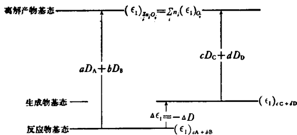
图 15-2. 反应物 ( aA + bB ), 生成物 ( cC + dD )
