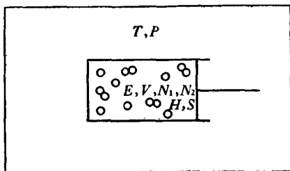
图 15-1. 反应体系与定压恒温介质构成的孤立体系
