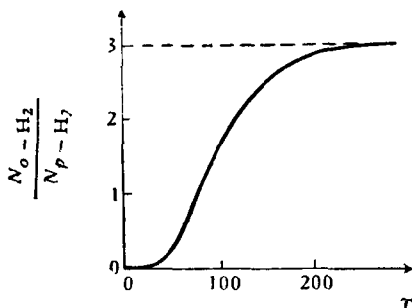
图 11-2. 轉化 p-H_2 \rightleftharpoons o-H_2 的平衡常数的温度曲线
