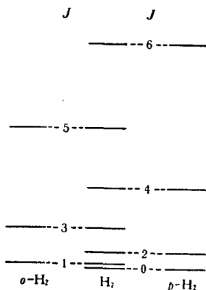
图 11-1. 正-氫、仲-氫和氫分子的核自旋-轉动状态示意图
