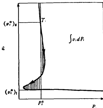
图 32-2. 根据范德华方程给出气体与液体在临界温度以下或 T_r < 1 时的平衡压力
