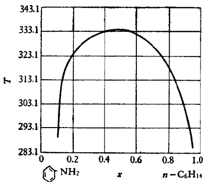
图 38-2. 苯胺和正己烷組成的二元体系的相图与临界混合現象
