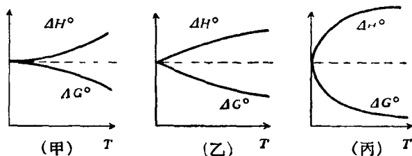
图 24-1. 化学反应的标准自由焓变 ( \Delta G^\circ ) 和标准焓变 ( \Delta H^\circ ) 在 0^\circ\text{K} 附近趋于一致的方式, 而 (甲) 是奈恩斯特在他著名的假说中肯定下来的一种方式。
