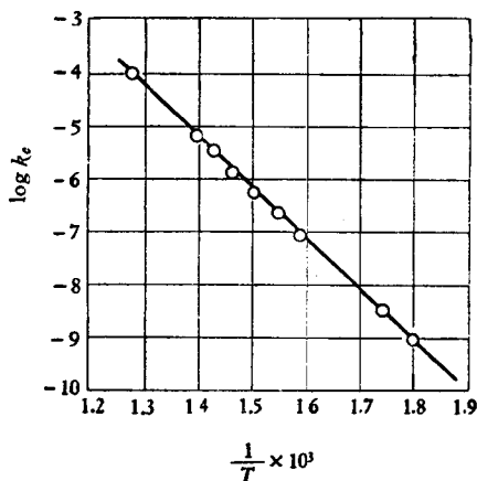
图 19-1. 反应 \text{HI} + \text{HI} \rightarrow \text{H}_2 + \text{I}_2 的图线 \log k_c - \frac{1}{T}
