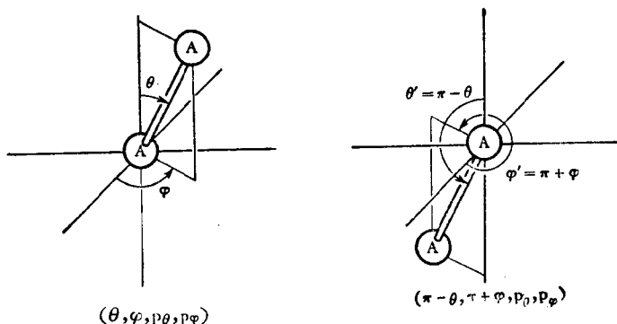
图 9-3. 代表同核双原子分子某一转动状态的两个相点： (\theta, \varphi, p_\theta, p_\varphi) 和 (\pi - \theta, \pi + \varphi, p_\theta, p_\varphi)
