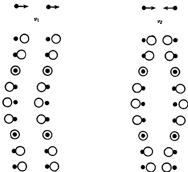
图 10-4. 单维偶合振子体系的两个简正振动方式
