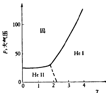
图 24-3. 液态 \text{He}^4 的凝固压力曲线
