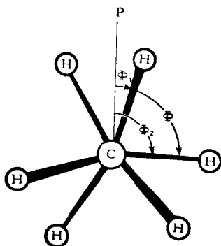
图 23-7. 乙烷分子中两个甲基的方位角坐标和內旋轉角坐标
