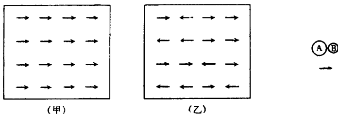
图 22-1. 不对称的双原子分子 AB 在晶体中的取向构型示意: (甲) 取向有序的构型; (乙) 取向无序的构型
