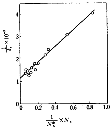
图 21-3. 二甲醚在 777.2° K 的分解反应及其速度常数的倒数 \frac{1}{k_r} 对浓度倒数 \frac{1}{N_A^*} 的图线
