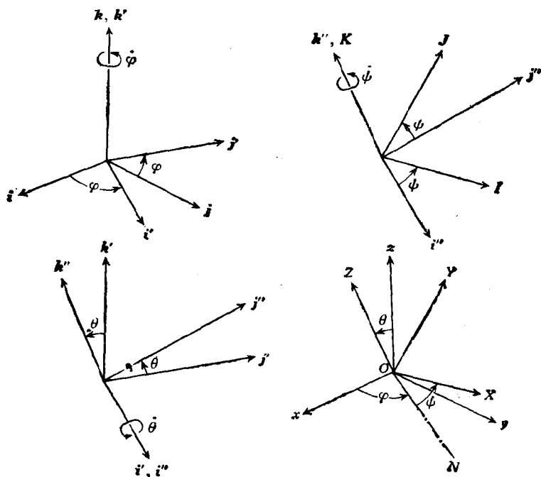
图 10-2. 欧勒角的定义
