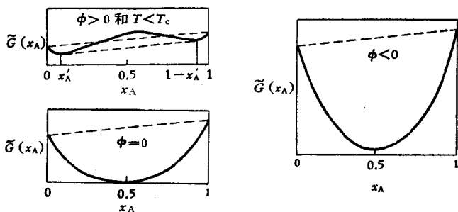
图 38-4. 若干具有代表性的 \tilde{G}(x_A) 曲线
