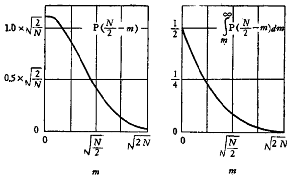
图 5-1. 可几率函数 P\left(\frac{N}{2} - m\right) 和定积分 \int_m^{\infty} P\left(\frac{N}{2} - m\right) dm
