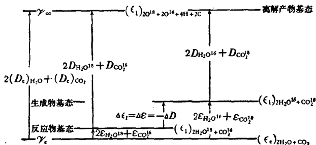
图 17-2. 同位素交换反应 2\text{H}_2\text{O}^{18} + \text{CO}_2^{16} \rightleftharpoons 2\text{H}_2\text{O}^{16} + \text{CO}_2^{18} 中反应物和生成物以及离解产物等基态的能值关联图
