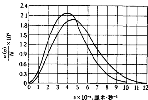
图 1-1. 氧气在 273 和 373°K 下的速度分布函数
