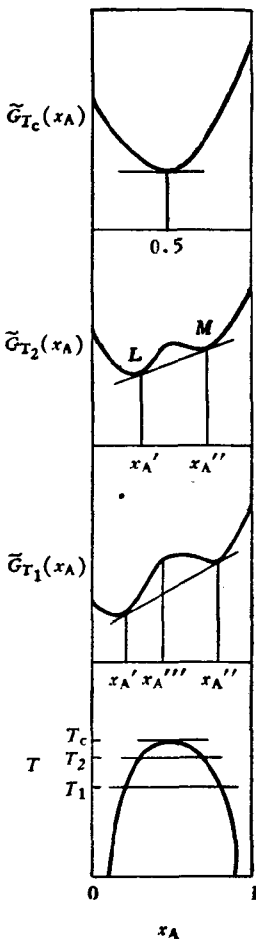
图 38-5. 給出二相区的 \tilde{G}(x_A) 曲綫
