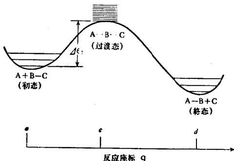
图 20-2. 反应体系 (A + B - C) 的位能函数沿反应坐标变化的情况
