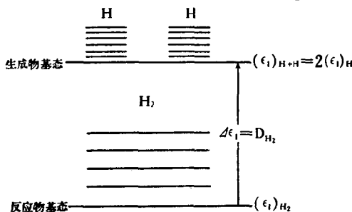
图 11-3. 一对氢原子( H + H )的能级示意图
