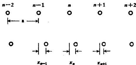
图 35-3. 一个单维点阵结构
