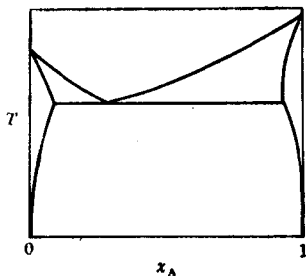
图 38-3. 拥有二固溶体相的合金体系 A-B 的相图例示
